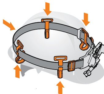
CASCO PROTECTOR Coloque los clips y las correas.
