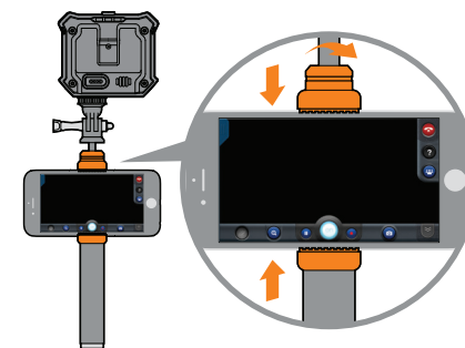
MONOPIÉ Coloque el soporte del teléfono y gire bloquear o desbloquear para ajustar la longitud del pie.
