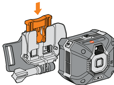
MONTURA PORTÁTIL Presione la palanca hacia abajo para un desenganche rápido.
